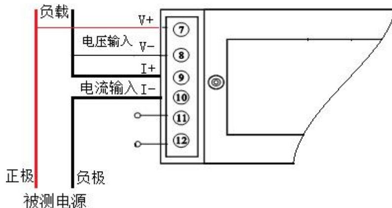
图 5.1、产品接线参考图
