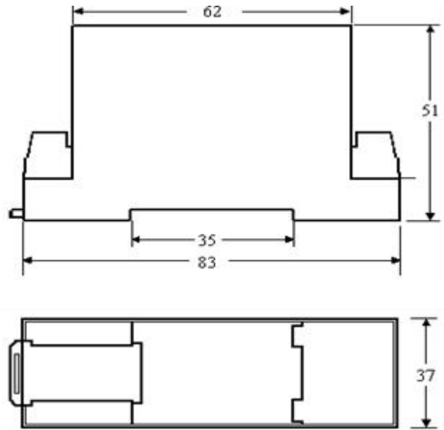
图 4.2、产品尺寸图（单位 mm）
